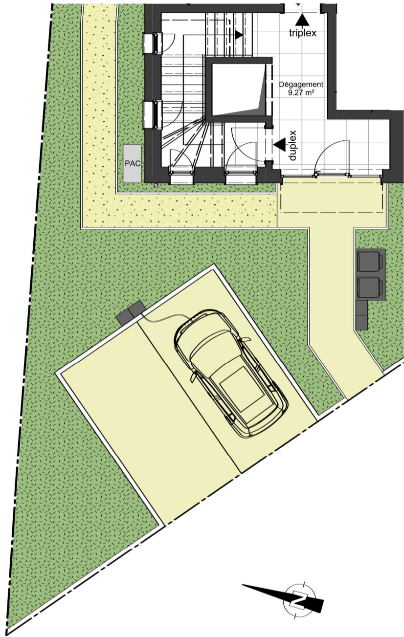
Rez-de-chaussée
