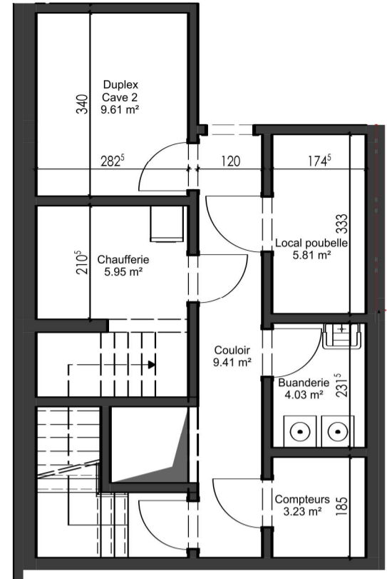
Sous-sol
